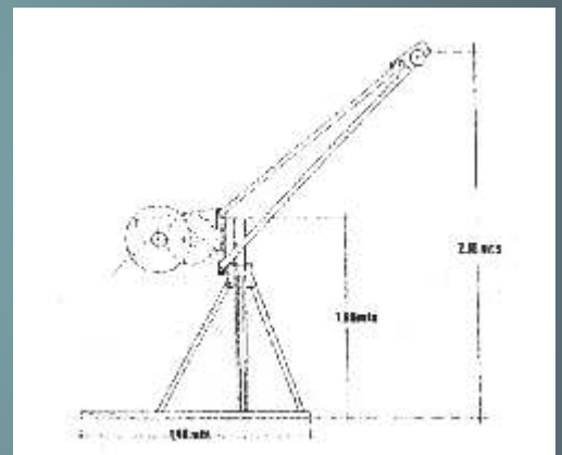
Pluma Grúa Modelo P-250 y P-300
